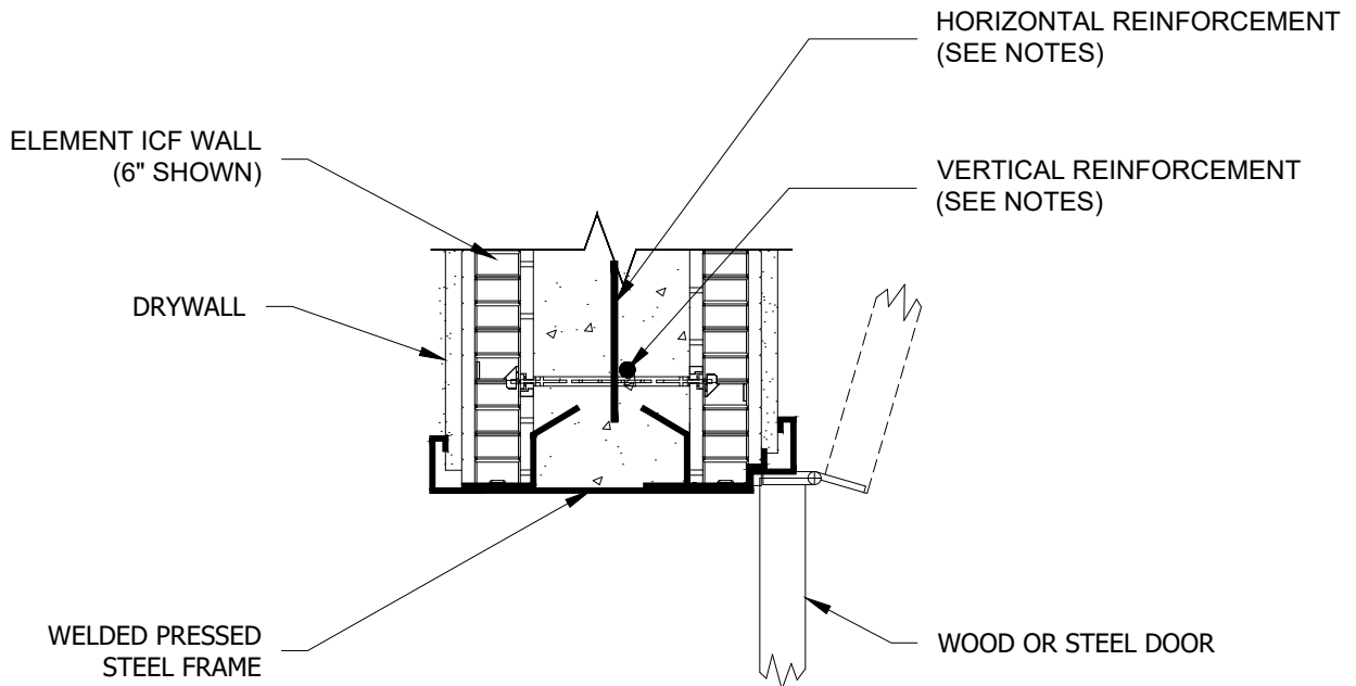
INTERIOR DOOR FRAME - JAMB FLUSH MOUNTED DOOR
